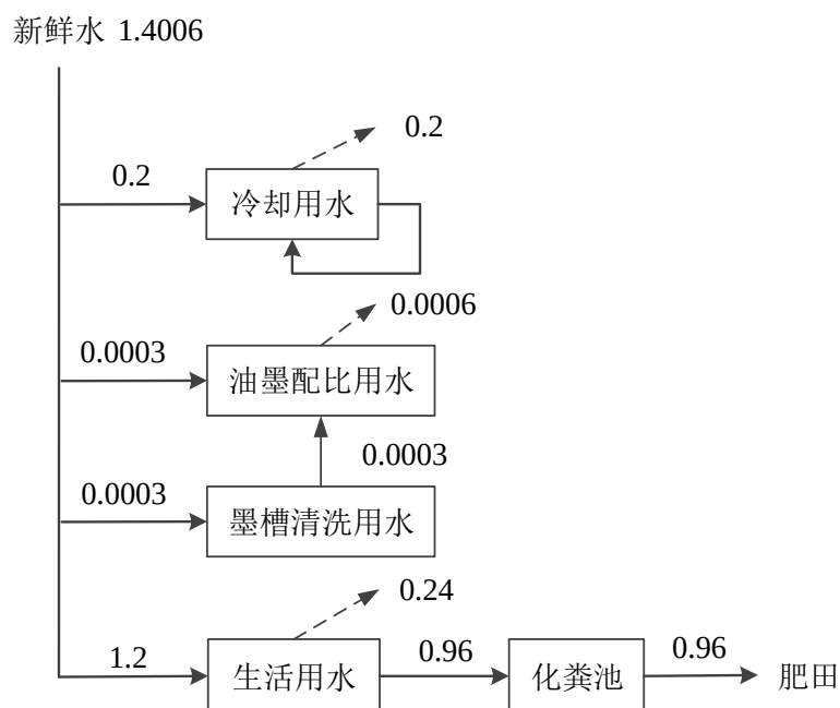
图 2-1 项目用排水平衡图 单位：m³/d
