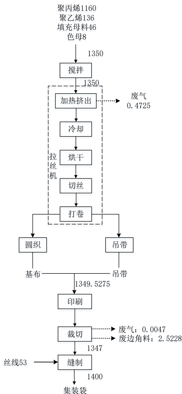
图 2-3 物料平衡图 单位: t/a
