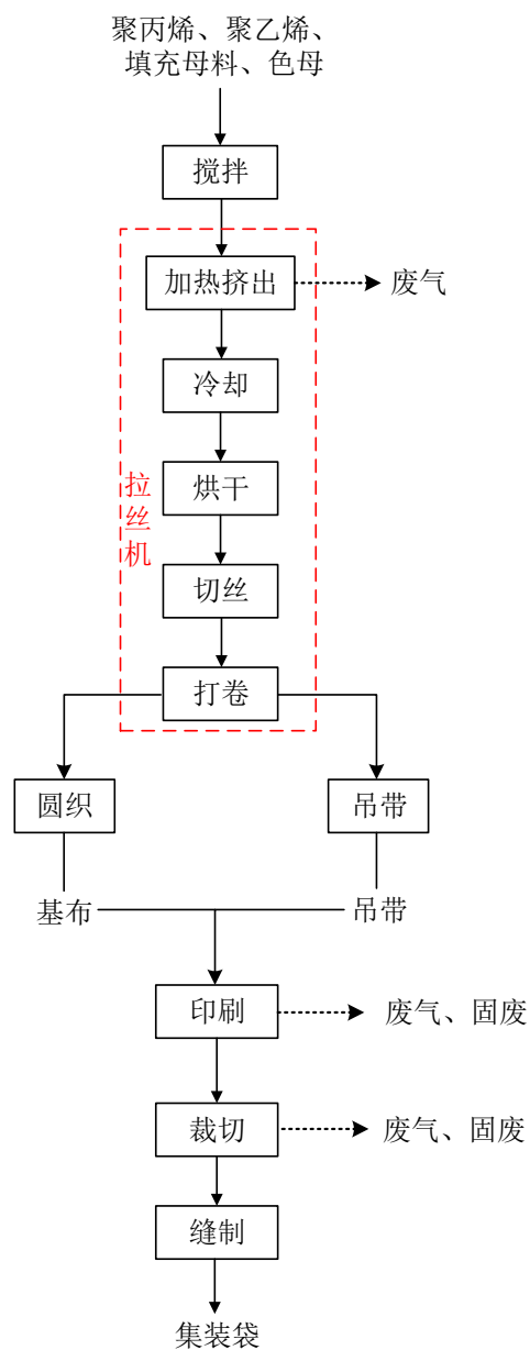
图 2-2 集装袋生产工艺及产污环节图
