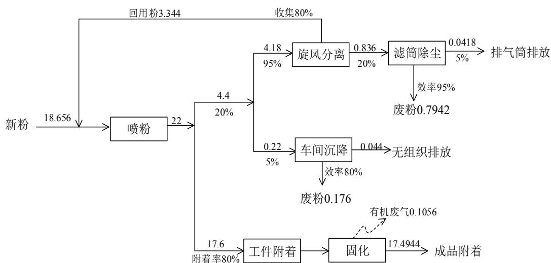
图 1 塑粉平衡图 单位:t/a
