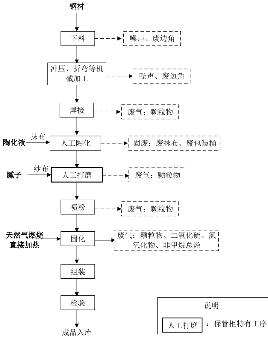
图2 工艺流程图
