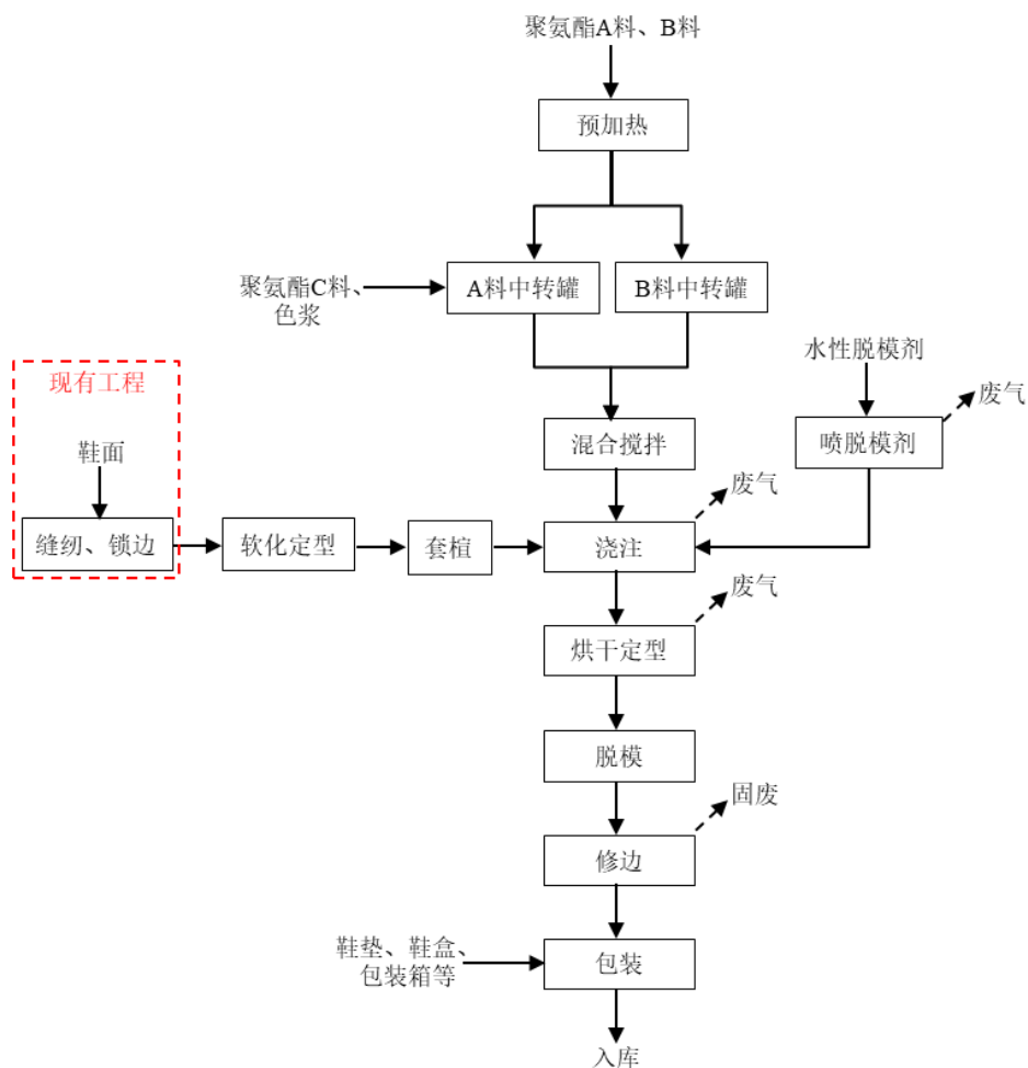
图 2-3 聚氨酯鞋底布鞋生产线工艺流程及产污环节图
